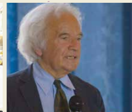
Duccio Demetrio
